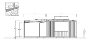
4. prospetto sud
