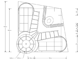
3. pianta, scala 1:50
