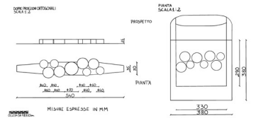
disegni tecnici in doppia proiezione ortogonale del prototipo scala 1:2
