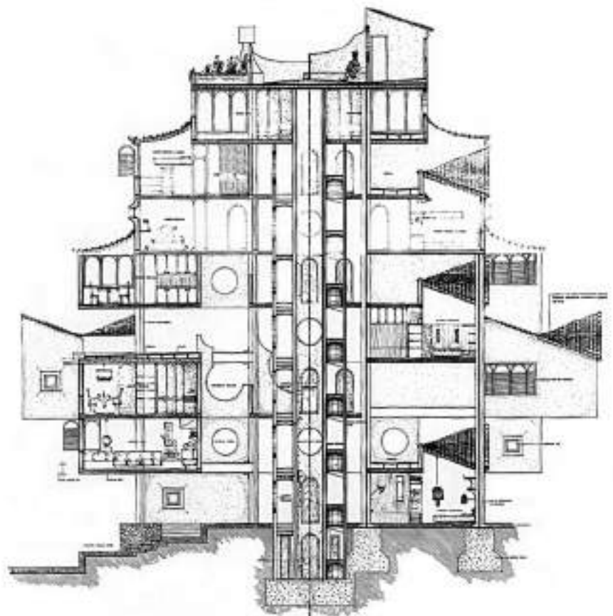
Ricardo Bofill, Xanadù, Alicante, 1971
