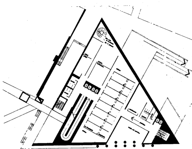
Gianugo Polesello, concorso per gli uffici per la camera dei Deputati, Roma, 1966 (secondo piano)
