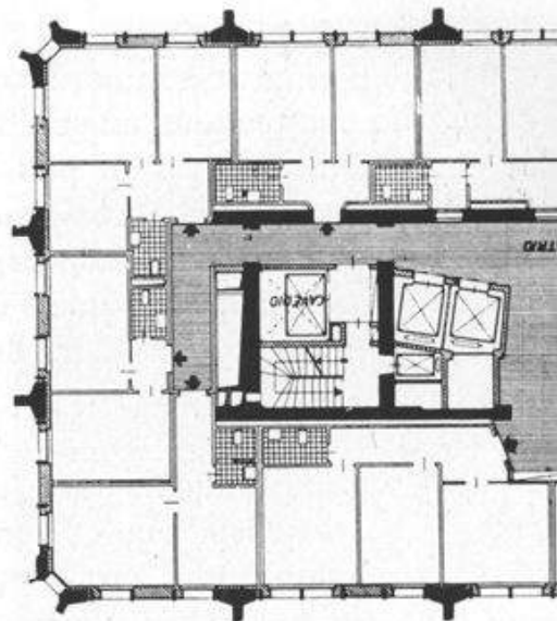
BBPR, Torre Velasca, Milano, 1955-1957
